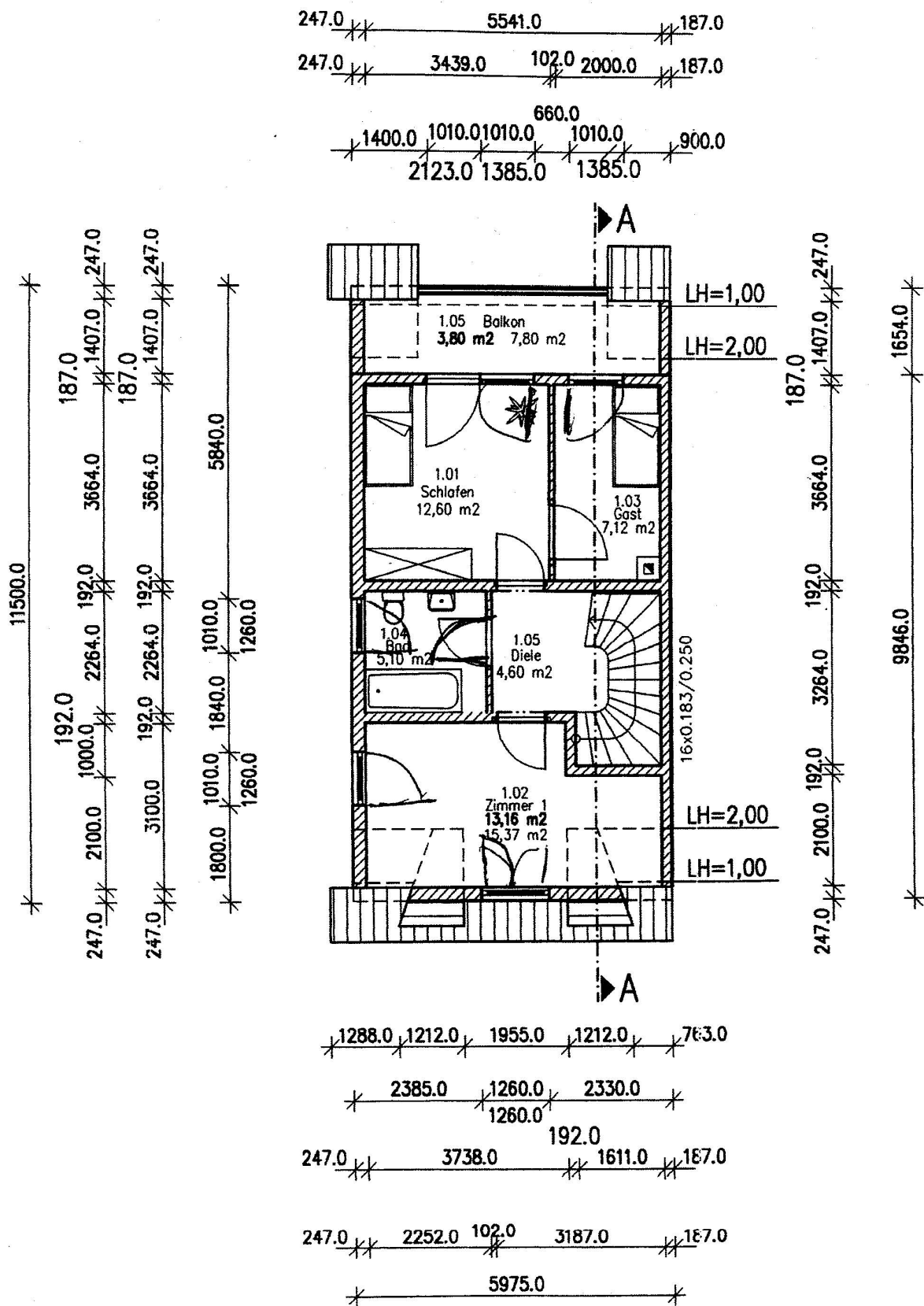
Grundriss Dachgeschoss
