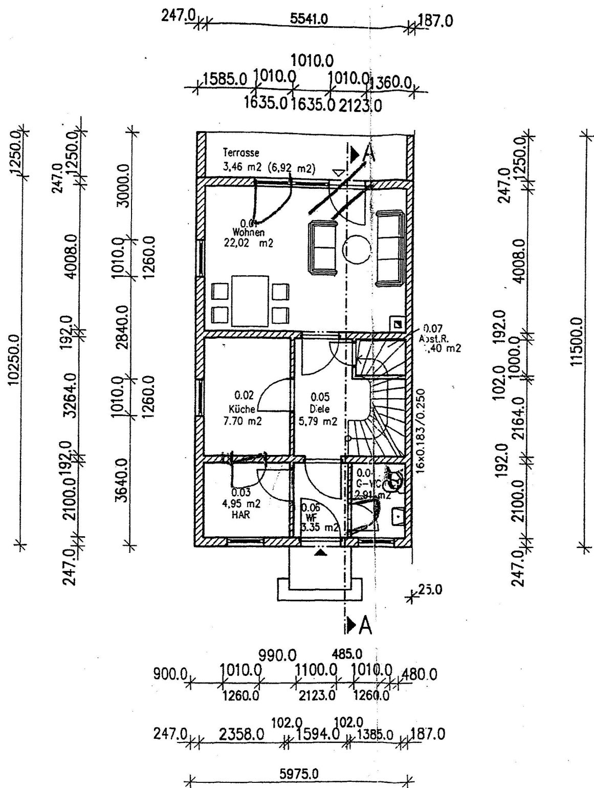
Grundriss Erdgeschoss
